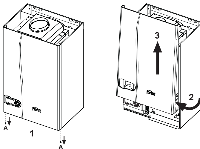
рис. 22 - Снятие кожуха
