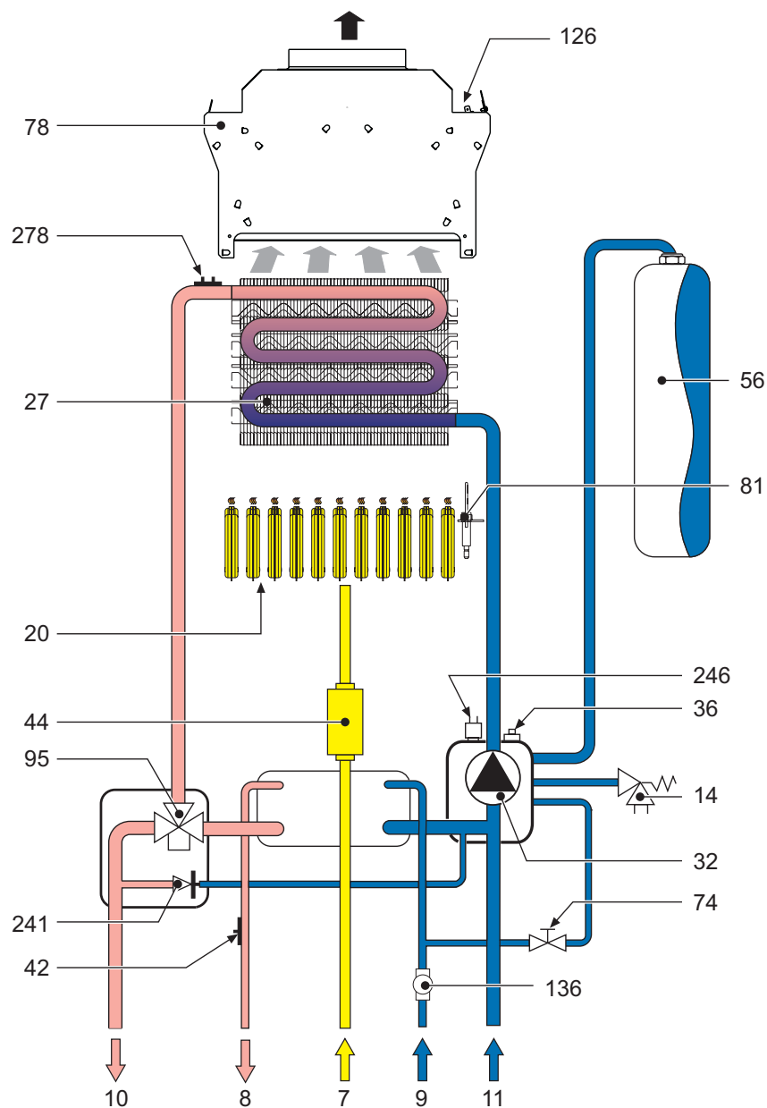
рис. 25 - Схема системы отопления и контура ГВС
