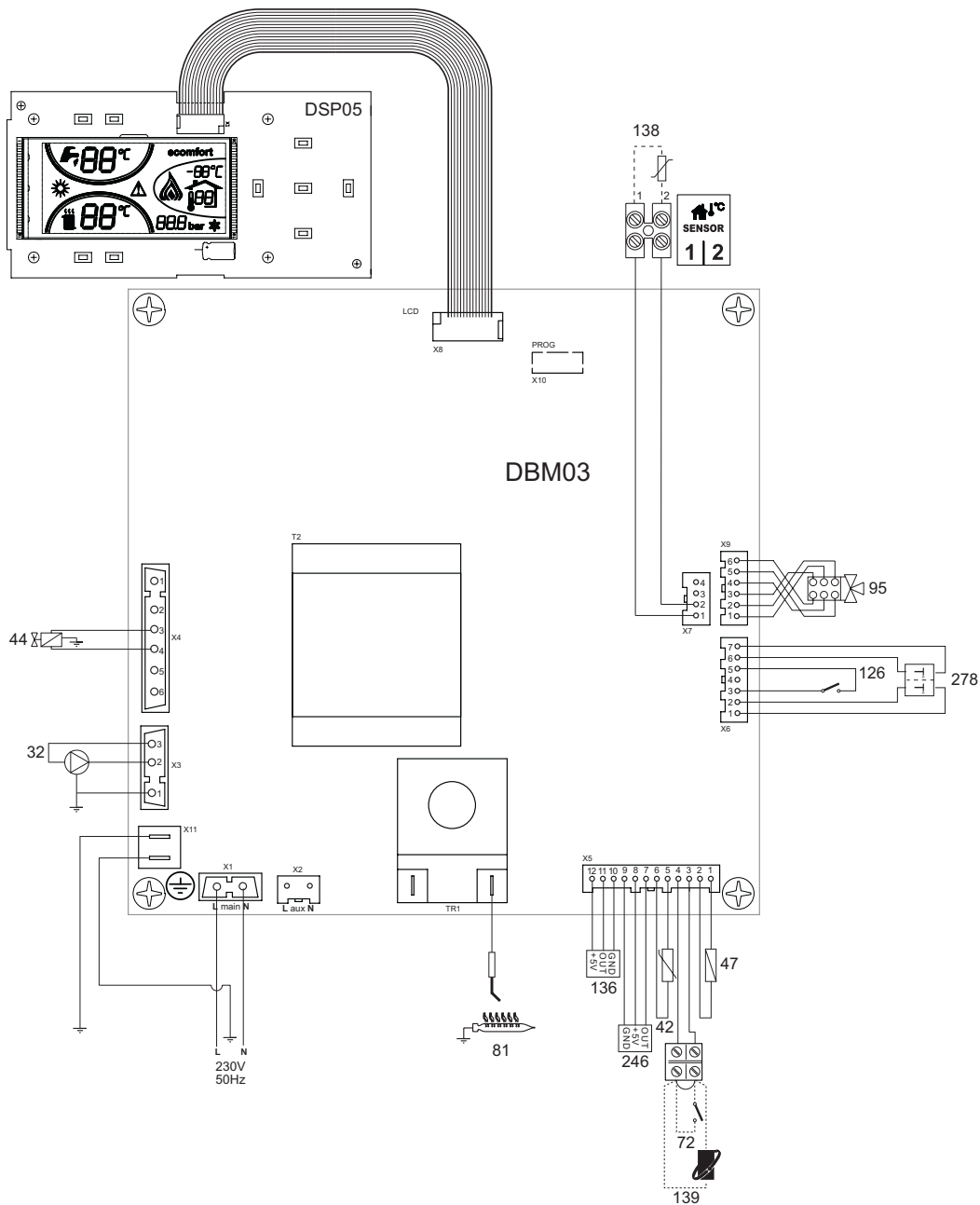
рис. 26 - Электрическая схема
